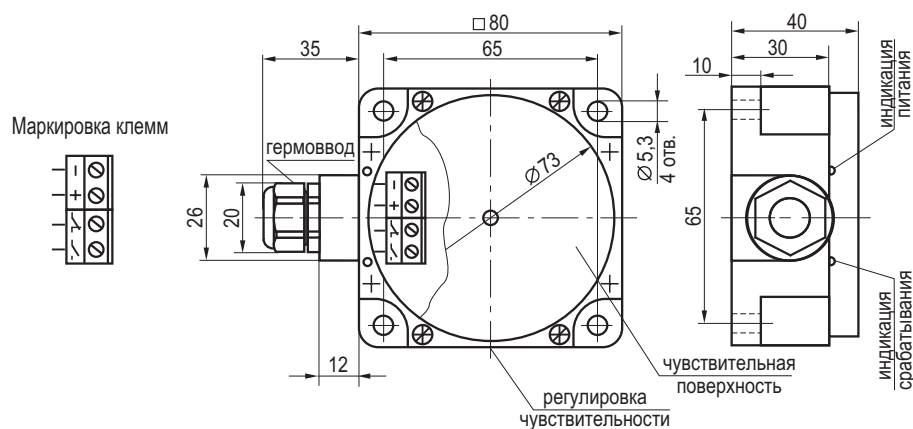
Габаритный чертеж
